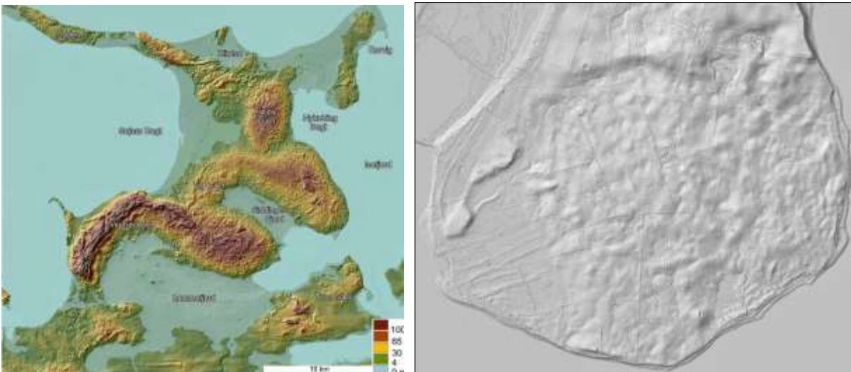
TV: De 3 Odsherredbuer, øverst Højby-buen, den ældste dannelse, derefter Vig-buen og sydligst Vejrhøj-buen, som er dannet som den sidste af de 3 buer. TH: Landskabet på Nakke viser en mulig moræne-rand op mod Maarbjerg højdedraget og typiske dødis-aflejringer i de mange lavninger, såkaldte dødishuller
